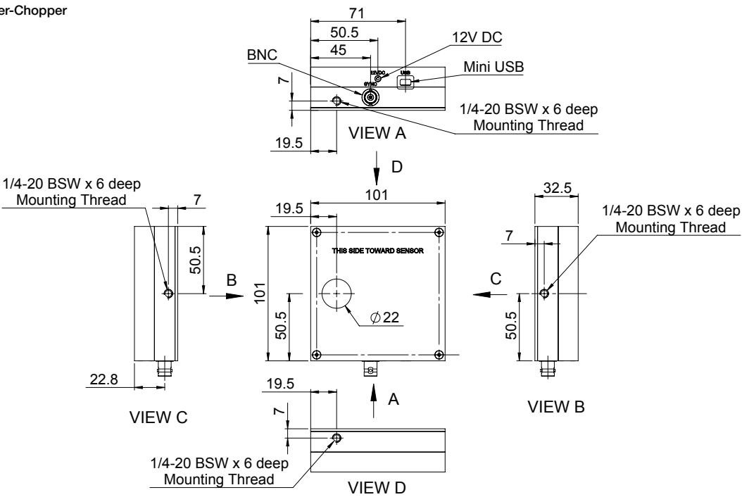
Radiometer-Chopper
