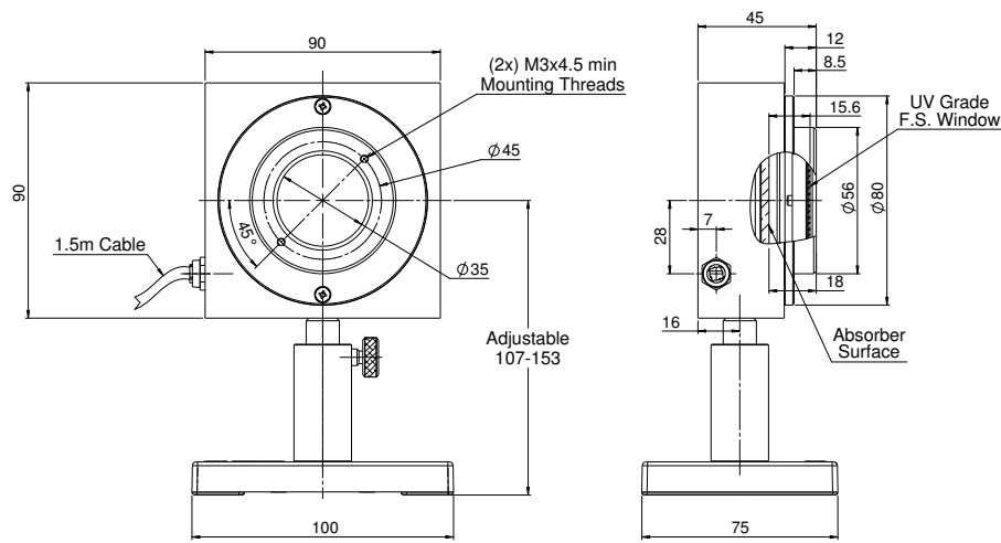
L40(500)A-LP2-DIF-35
