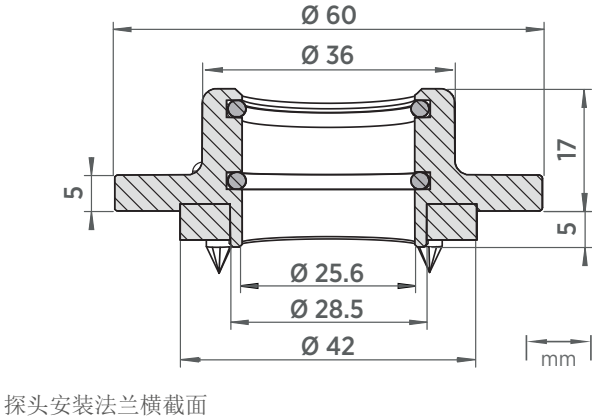
探头安装法兰横截面
